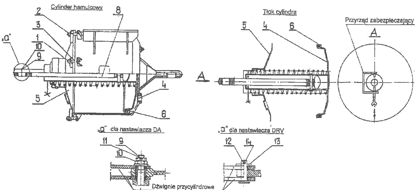
Rys. nr 18. Wymiana pierścienia uszczelniającego tłok cylindra.
